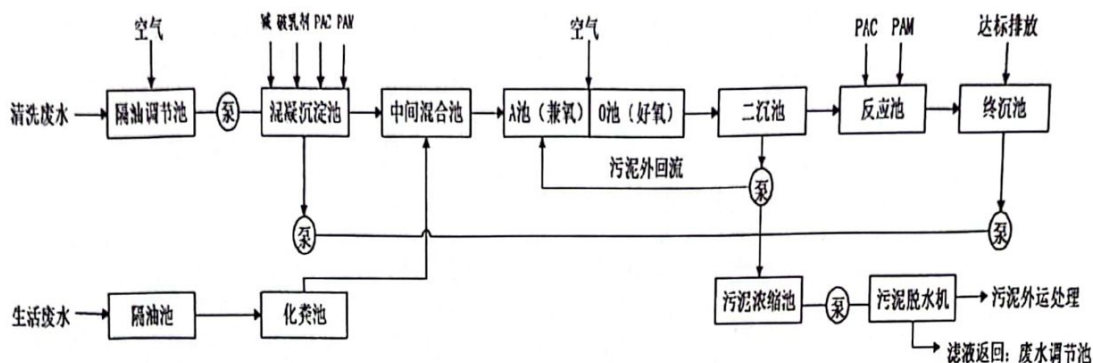
图1 项目实际废水处理工艺流程图
